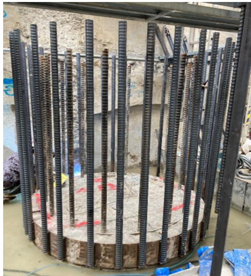
開先付き鉄筋 現場使用例
