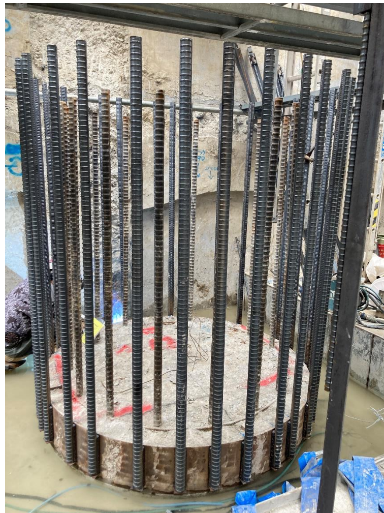
開先付き鉄筋 現場使用例
